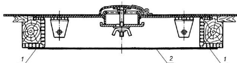
Рис. 8.2. Заделка печной разделки бумагой: 1 — место приклеивания; 2 — бумага.
