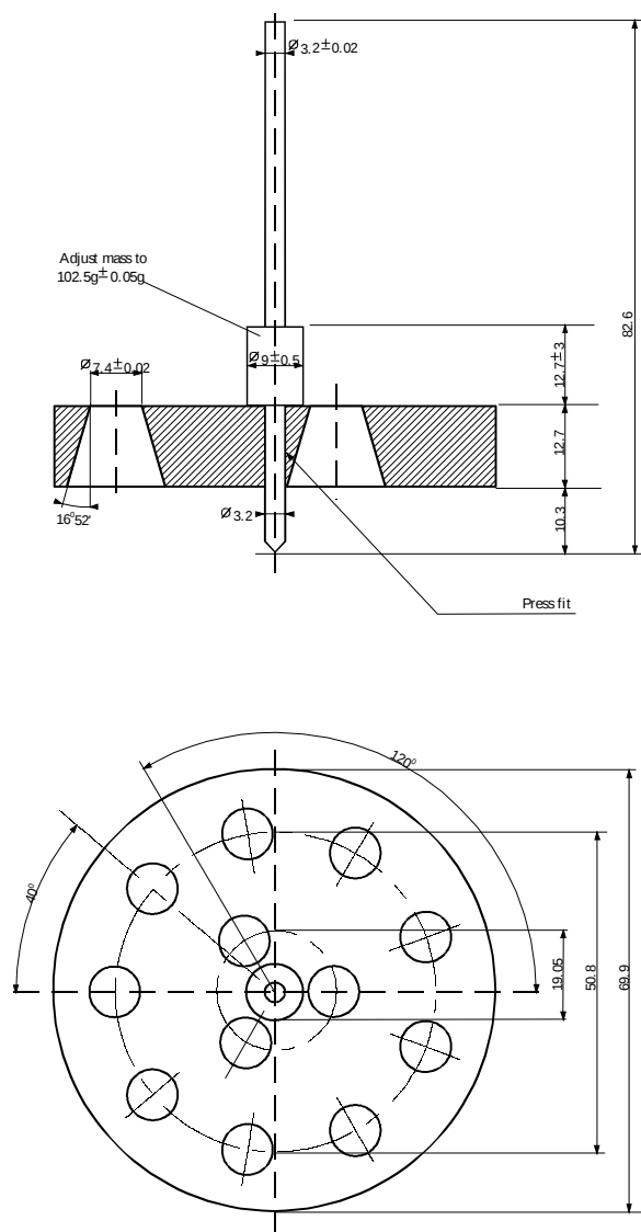
Рис. 2.4. Пенетрометр
