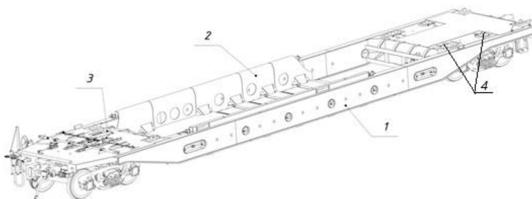
Рисунок 5б – Платформа модели 13-6701
