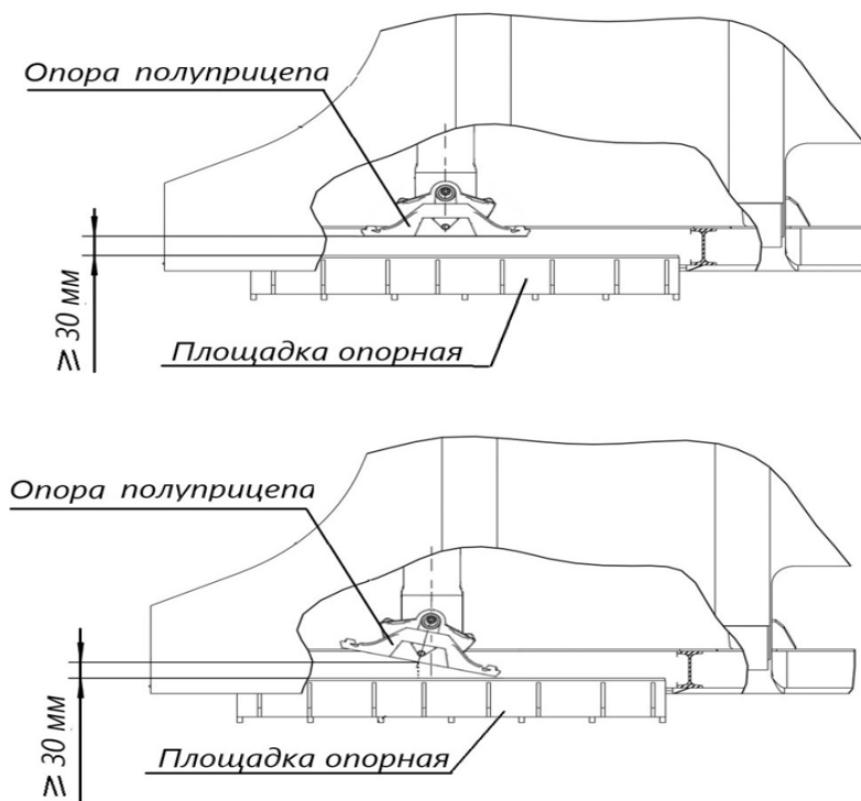
Рисунок 42 – Схема контроля положения опор полуприцепа
