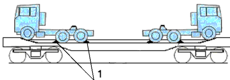
Рисунок 18 – Размещение и крепление тягачей а – одного тягача; б – двух тягачей; 1 – колесный упор
