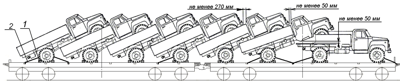
Рисунок 19 – Размещение и крепление автомобилей на сцепе платформ 1 – упорный брус от продольного смещения; 2 – растяжка
