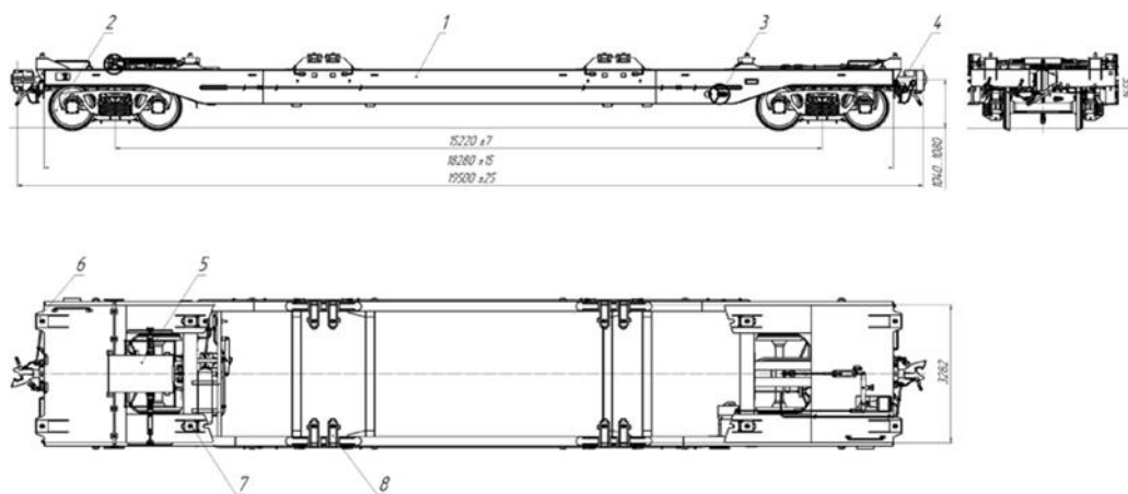
Рисунок 5 – Платформа модели 13-6987
