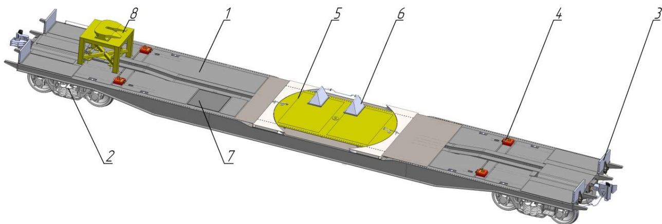
Рисунок 5а – Платформа модели 13-9938
