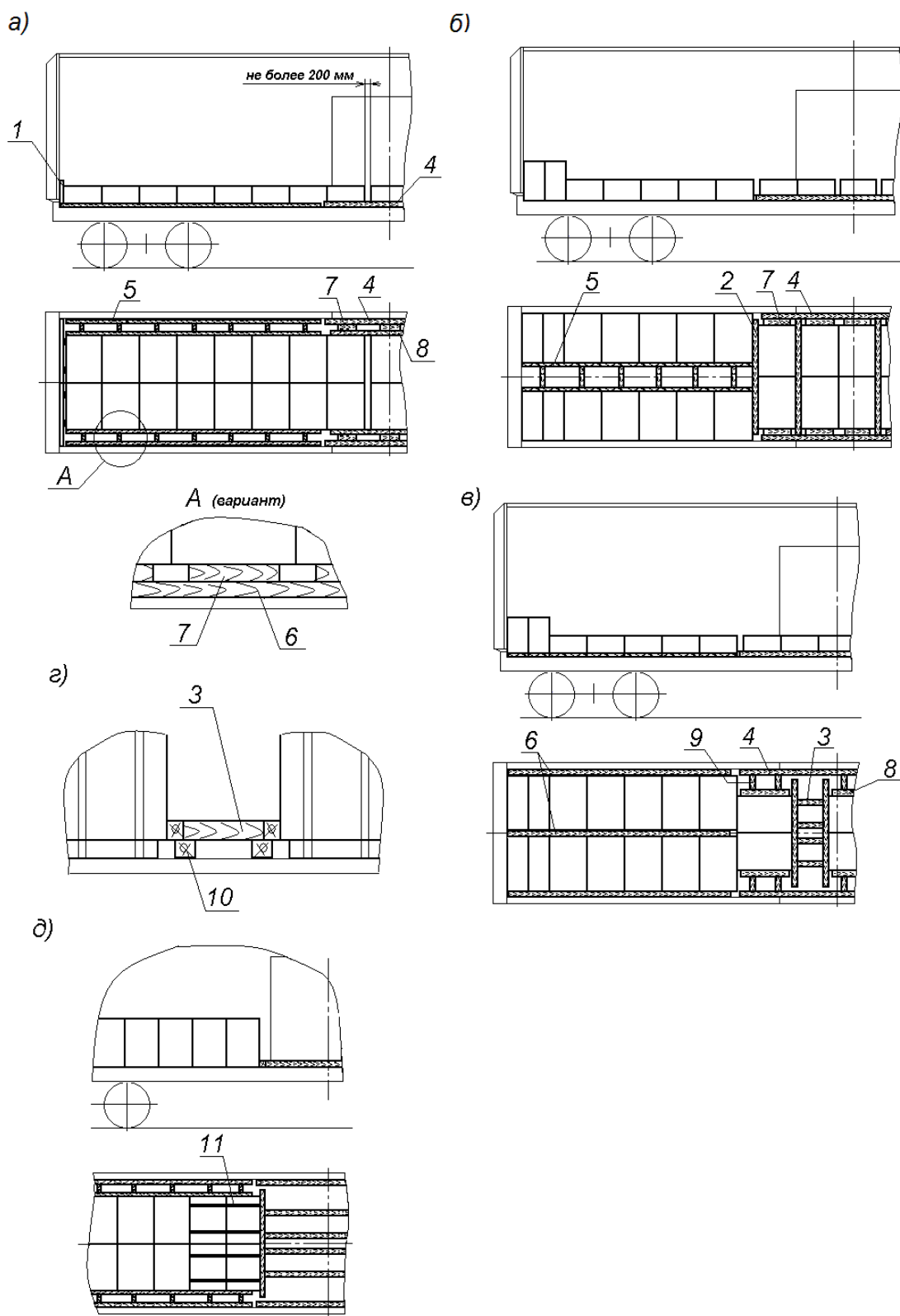
Рисунок 25 – Примеры размещения и крепления пакетов цветных металлов
