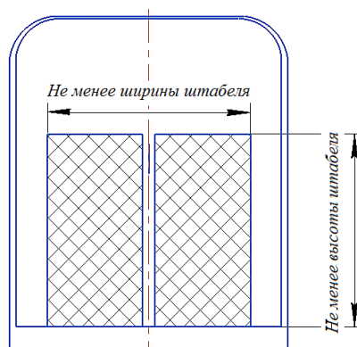
Рисунок 42 – Схема установки сотовых панелей для ограждения торцовых стен крытого вагона
