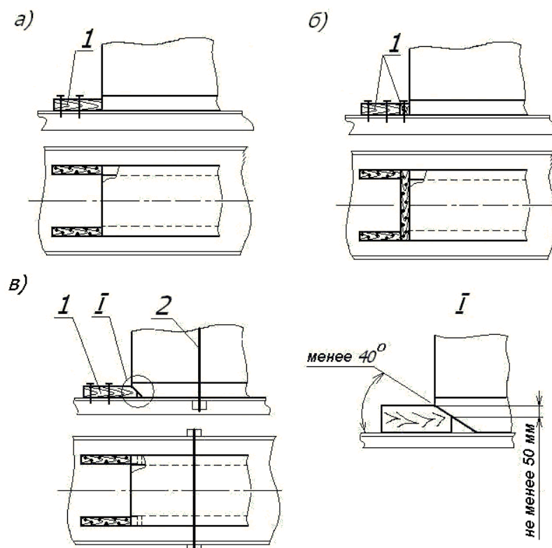
Рисунок 8 – Примеры крепления груза на салазках в продольном направлении брусками:
