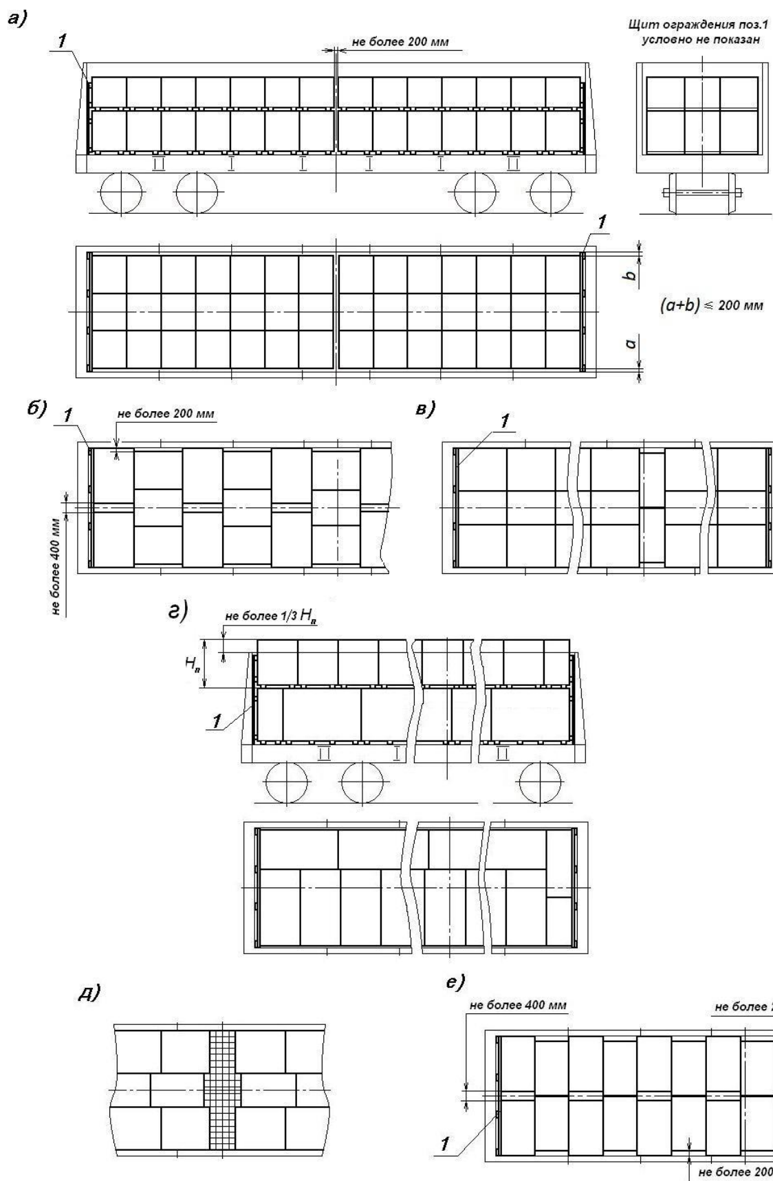
Рисунок 3 – Примеры размещения пакетов 1 – щит ограждения дверей
