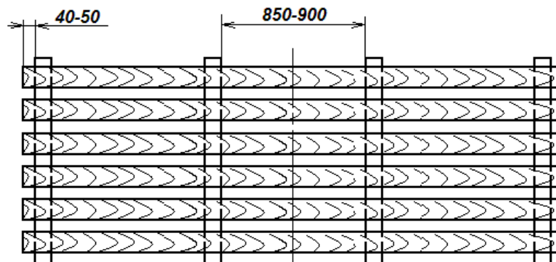
Рисунок 2 – Щит ограждения
